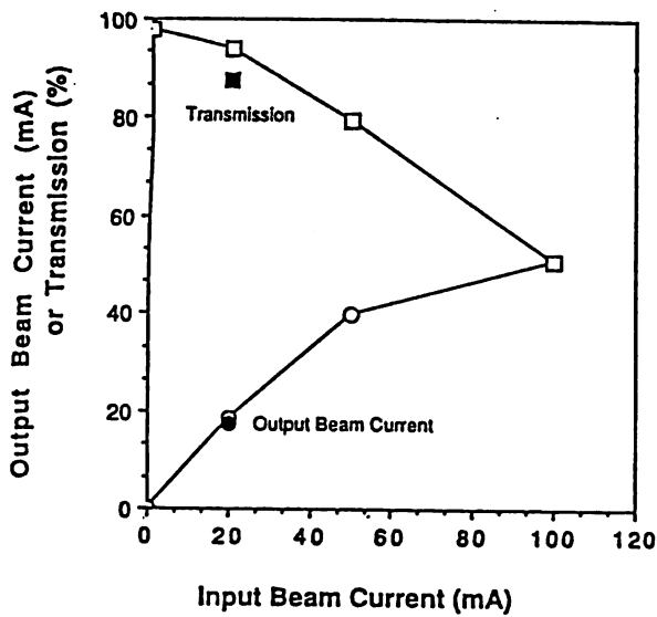
図4 PARMTEQ を用いたシミュレーションで得られた、入力ビーム電流と出力ビーム電流及び透過効率の関係 ○□:入力ビームエミッタンス=1.5 \pi *mm*rad ⊙⊠:入力ビームエミッタンス=2.3 \pi *mm*rad
