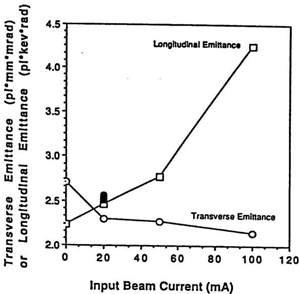
図5 PARMTEQ を用いたシミュレーションで得られた、入力ビーム電流と出力ビームのエミッタンスの関係 ○□:入力ビームエミッタンス=1.5 \pi *mm*rad ⊙⊠:入力ビームエミッタンス=2.3 \pi *mm*rad
