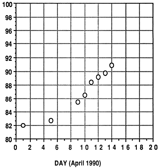
Fig. 2 修正によるベクトル化率の増加。
