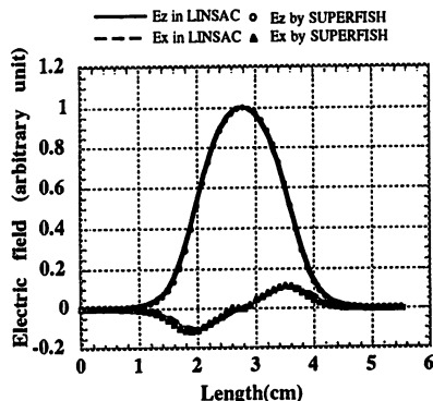
図1 ユニットセルの電場分布の例。LINSAC 中の近似値と SUPERFISH の計算結果を示す。
