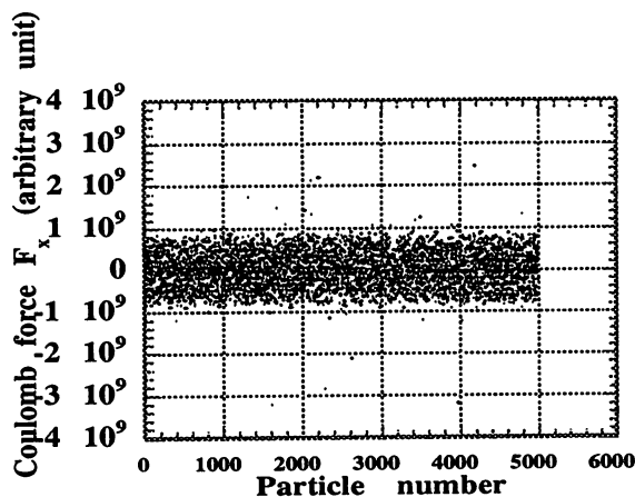
図8 計算途中の第2924ステップにおける 全粒子 (5000個) のx方向のクーロン力。1ステップは高周波位相に換算して約2°。本図は、平均的な、セルの中のクーロン力を表すと考えられる。
