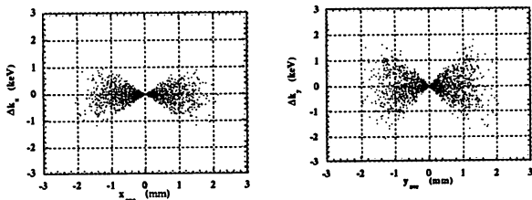
図3 あるユニットセルを通過した時の横方向の運動エネルギーの変化を、そのセルの平均横座標に対して図示。磁場勾配がオンの場合。
