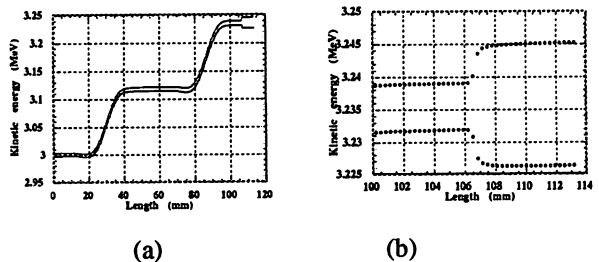
図5 (a) 第1と2セルを通過した時の2個の粒子の縦方向の運動エネルギーの変化。位置107 mm付近で衝突によるエネルギー変化が見られる。 (b) 左図を拡大した図。
