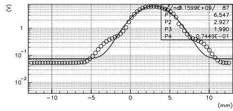
調整後
